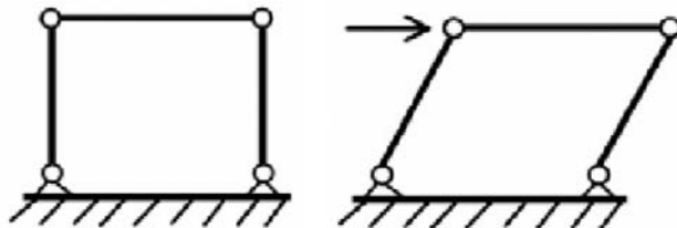
Struttura labile
