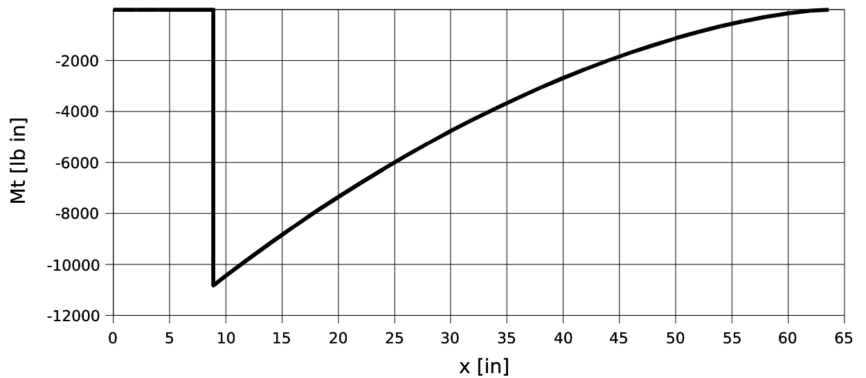
Momento torcente
